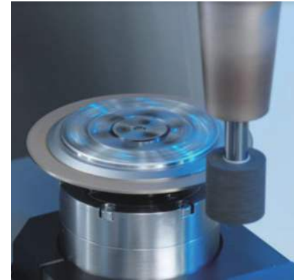
砂轮修整器
